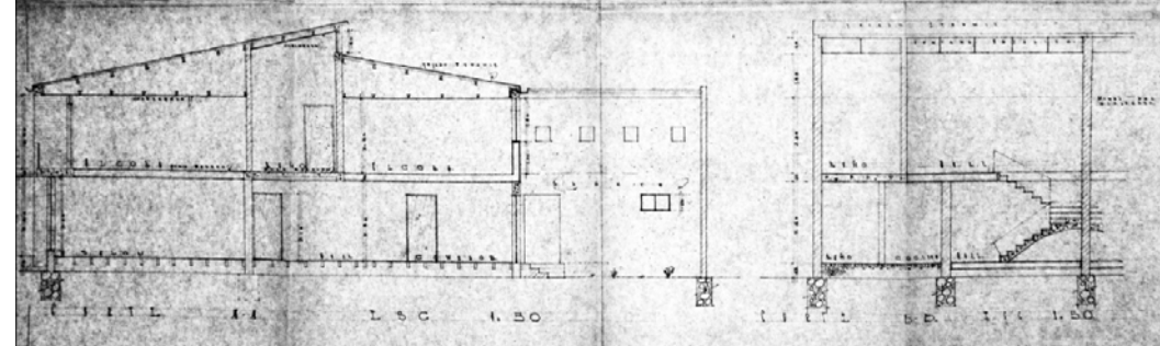
CORTE LONGITUDINAL
